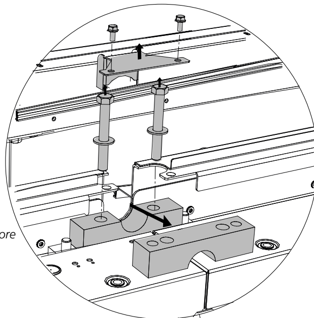
Staffe di montaggio dell'albero
