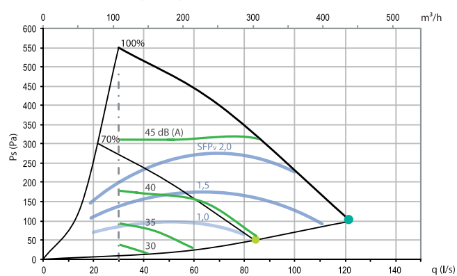
Débit d'air et niveau de puissance sonore en périphérie
