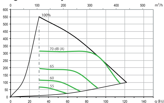
Niveau de puissance sonore à la gaine d'air rejeté
