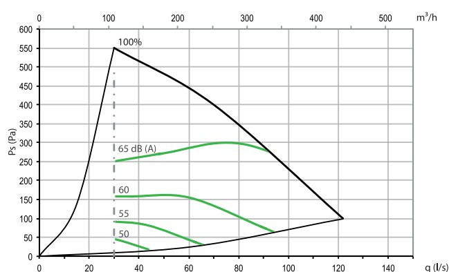
Niveau de puissance sonore à la gaine d'air extrait
