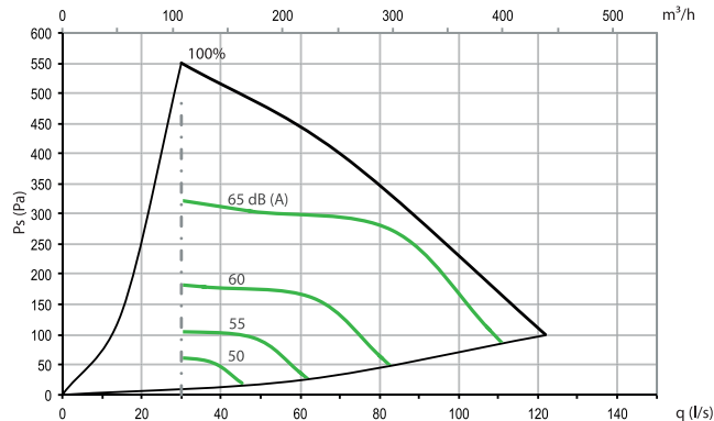
Niveau de puissance sonore à la gaine d'air extérieur
